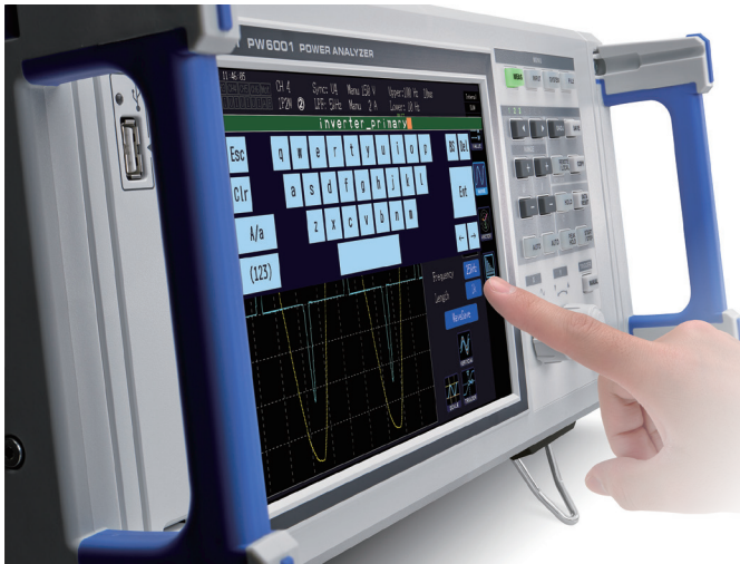
소프트웨어 키보드를 탑재한 9인치 터치패널
