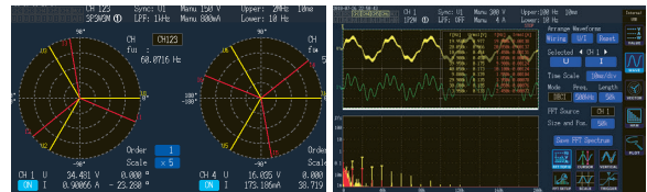
입력파형의 FFT 해석에 의한 노이즈 측정, 출력의 고조파 측정이 가능
