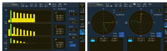
고조파 막대 그래프 표시
