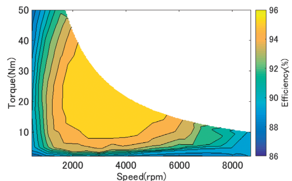
MATLAB 에 의한 효율 맵 표시 예
