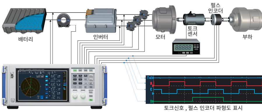
토크신호, 펄스 인코더 파형도 표시
