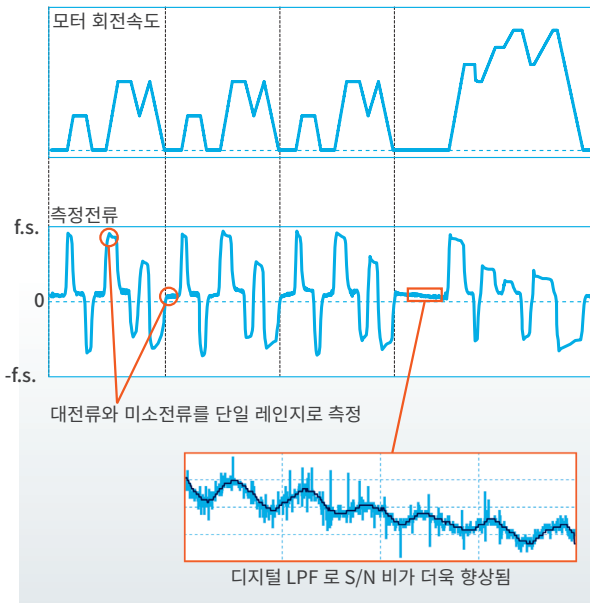
모터 계속 시의 변환효율을 레인지 전환 없이 측정
