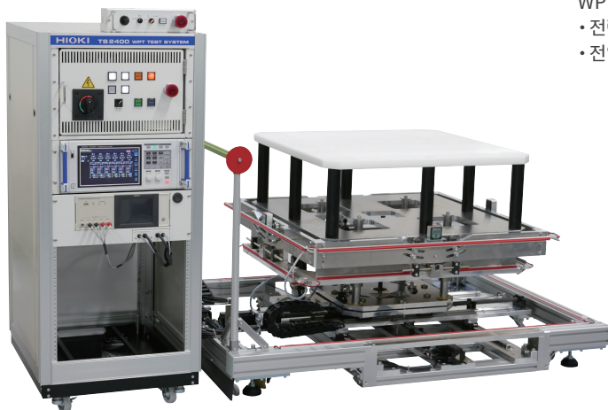
WPT 평가 시스템 TS2400
