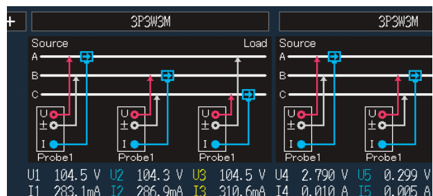
결선실수를 방지하는 결선확인기능
