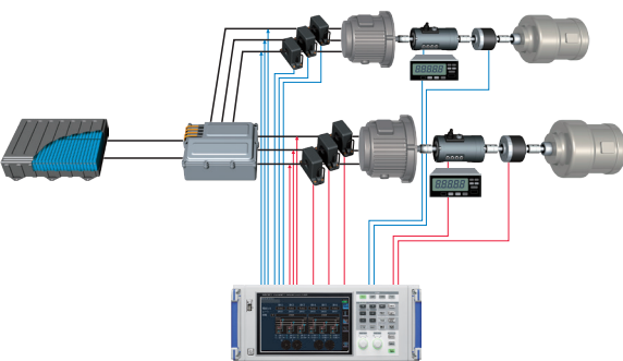
2 개의 모터 측정 예
