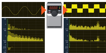
인버터 입출력, 각각의 기본파에 동기
